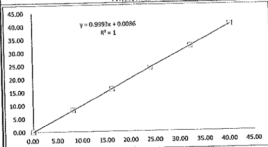
高濃度檢量線圖
