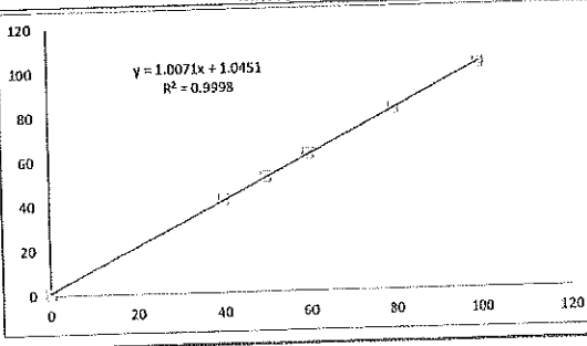
低濃度檢量線圖
